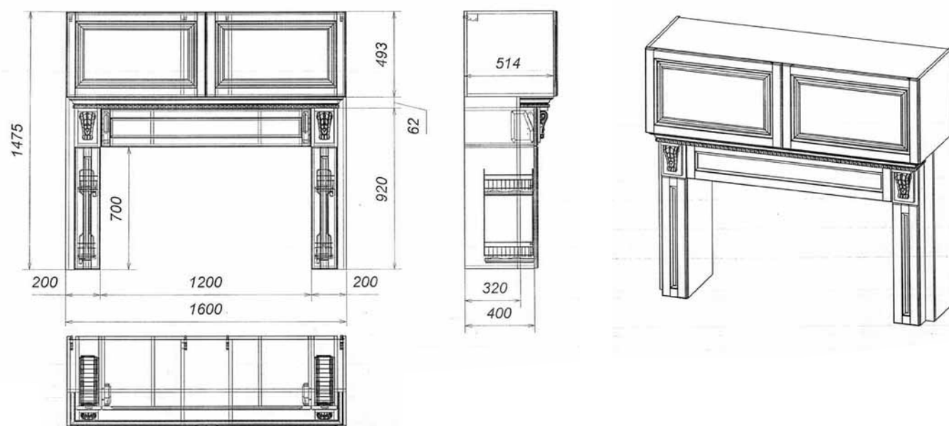
Габаритные размеры портала 3
