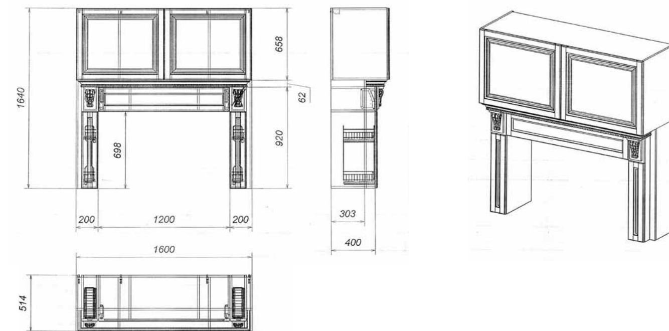
Габаритные размеры портала 3.1
