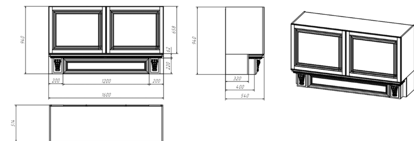
Габаритные размеры портала 3
