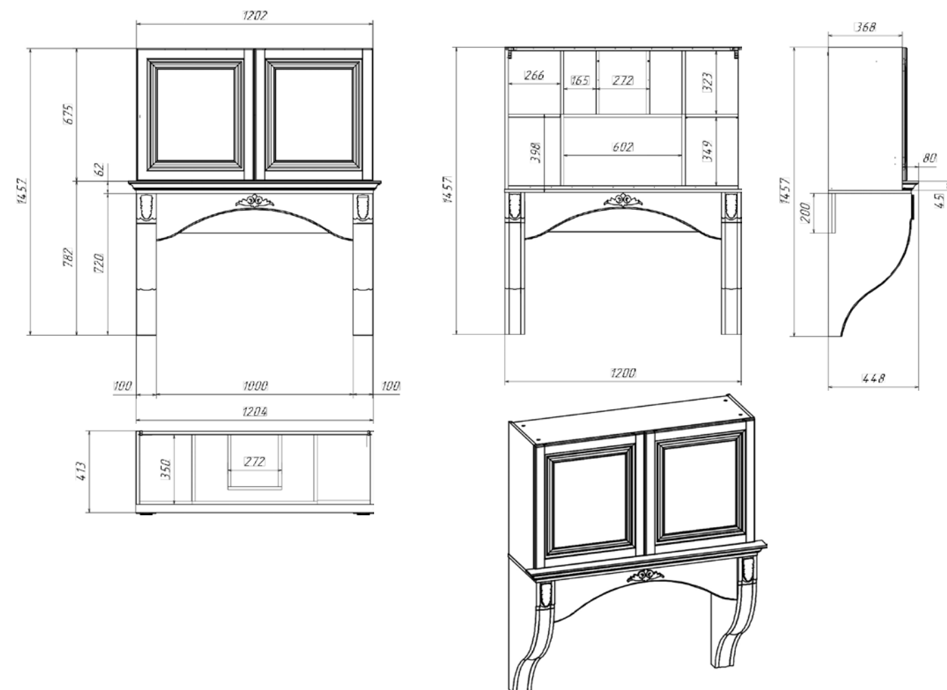
Габаритные размеры портала 1
