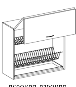
В600КРП, В700КРП, В800КРП
