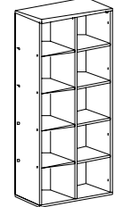
Шкаф П034.12С: L914xВ443xH2105
