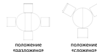
Стол «Верди 12А» П318.07: L1100/1450xВ1100xH778
