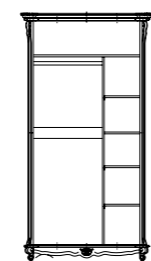
Шкаф ПЗ49.24: L1240xВ696xH2258
