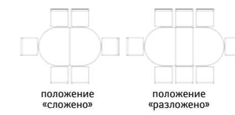
Стол «Валенсия 18» П394.03: L1800/2300xВ1100xН762
