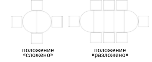
Стол «14А» П323.12: L1300/1770/2240/2710xВ1000xH778
