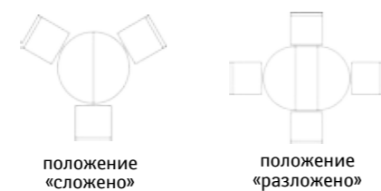
Стол «Верди 11/1» П317.04: L800/1100xВ800xH778
