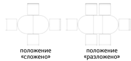
Стол «Верди 5РД» П106.16: L1380/1780xВ800xH740
