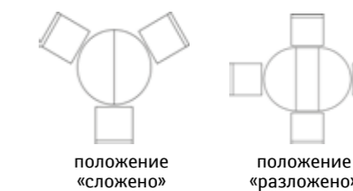
Стол «Валенсия 11» П358.07: L1000/1350xВ1000xН778
