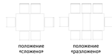
Стол «Кармен» (раздвижной) ПЗ.581.0.10: L1600/2100xB900xH777
