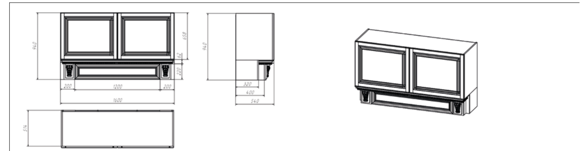
ГАБАРИТНЫЕ РАЗМЕРЫ ПОРТАЛА 3.1
